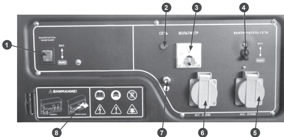
Рис. 3 Панель управления
