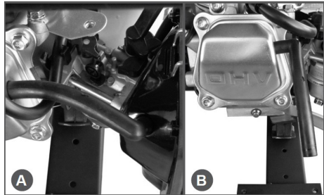
Рис. 11 Трубка сапуна
